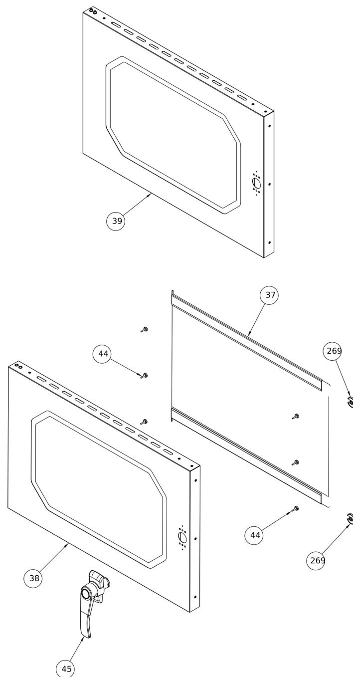
Door
